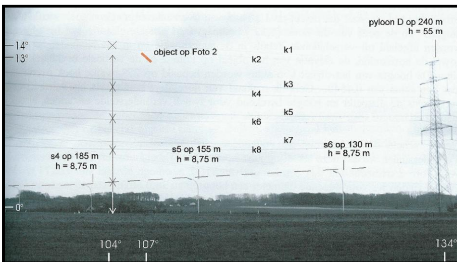
Fig. 16: Meting van de hoogte van de kabels tussen pyloon B en pyloon D op het punt waardeze de N437 kruisen (azimut = 104°, hoogte = 14°). Het hoogste kabelpaar bevindt zich ongeveer 5,3 maal hoger als de straatlampen op dit punt van de weg. © CAELESTIA
